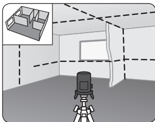
CZ / Příklady použití nivelačního laseru, obr. 2 SK / Príklady použitia nivelačného lasera, obr. 2 HU / A keresztlézer felhasználási példái, 2. ábra DE / Anwendungsbeispiele vom Nivellierlaser, Abb. 2 EN / Example of use of the levelling laser, Fig. 2
