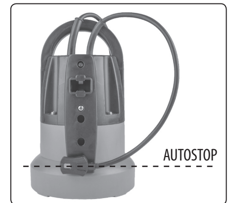
Abb. 4b, Drehung des Füllstandssensors entsprechend der Position der Öffnung
