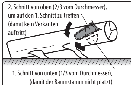
Baumstamm an einem Ende abgestützt, Abb. 19
