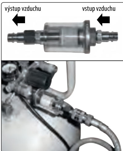
Obr. 8, pripojenie filtra (odlučovača) Extol® Craft 8865101
