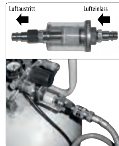
Abb. 8, Anschluss vom Filter (Abscheider) Extol® Craft 8865101
