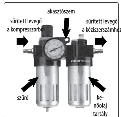
10. ábra. Extol® 8865105 levegő előkészítő egység
