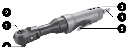
Obr. 2, račňový utáhovač Fortum®4795015
