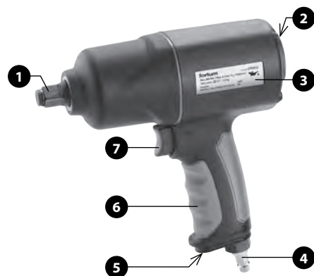
1. ábra. A 4795012 típusú ütvecsavarozó részei
